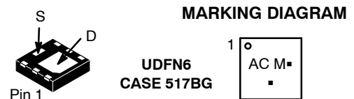
P-Channel MOSFET
