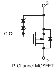
P-Channel MOSFET
